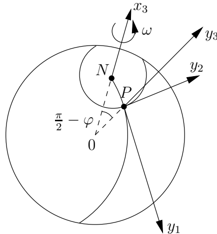
Abbildung 1: Darstellung des \mathbf{y} -Koordinatensystems für das Foucault'sches Pendel.
